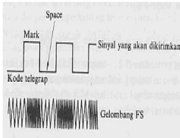
Gambar 5.7 Sinyal FS
